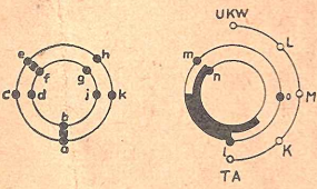
Schalter am linken Anschlag (Schaltstellung „UKW“)
